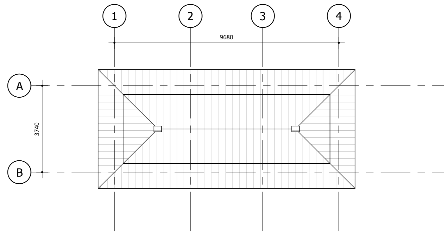
1e verdieping bestand
