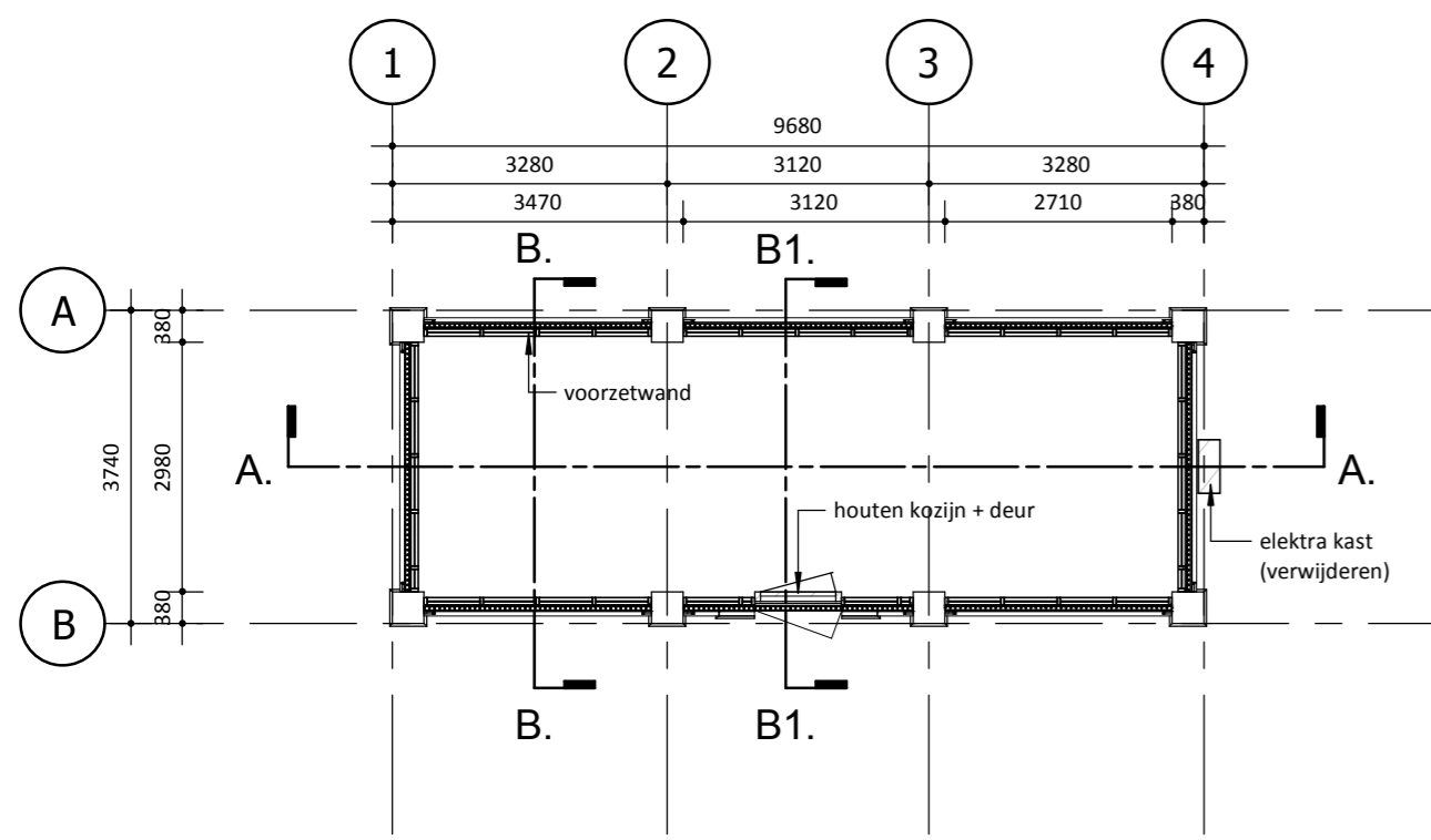
begane grond bestand
