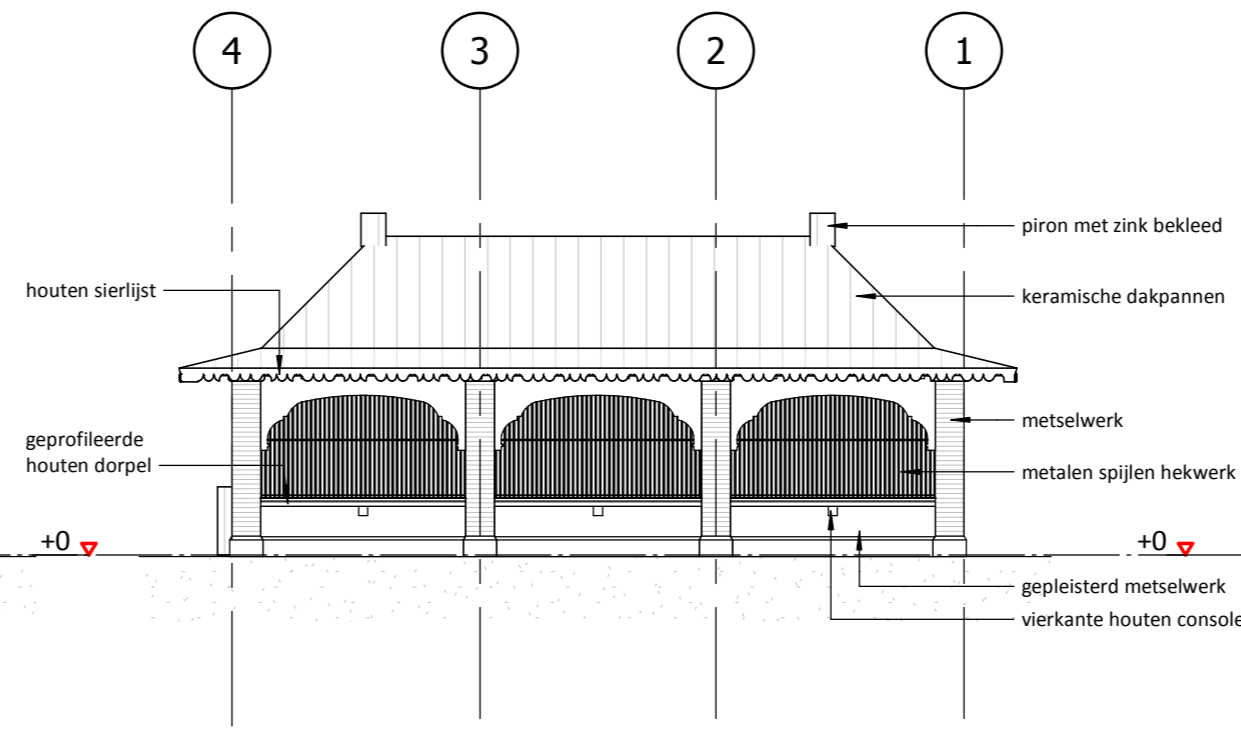
achtergevel bestand
