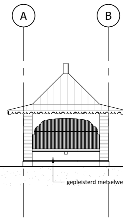
linkergevel bestand
