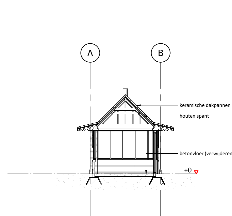
doorsnede B1 bestand
