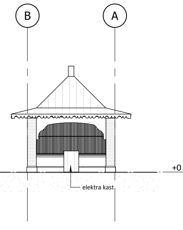
rechtergevel bestand
