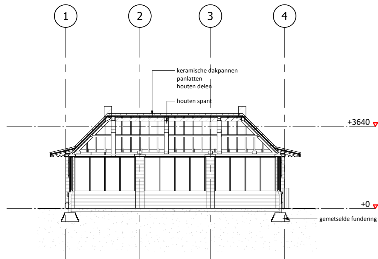
doorsnede A bestand
